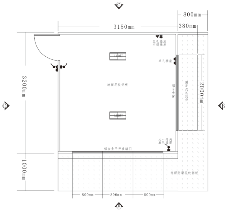
门卫岗亭平面图
