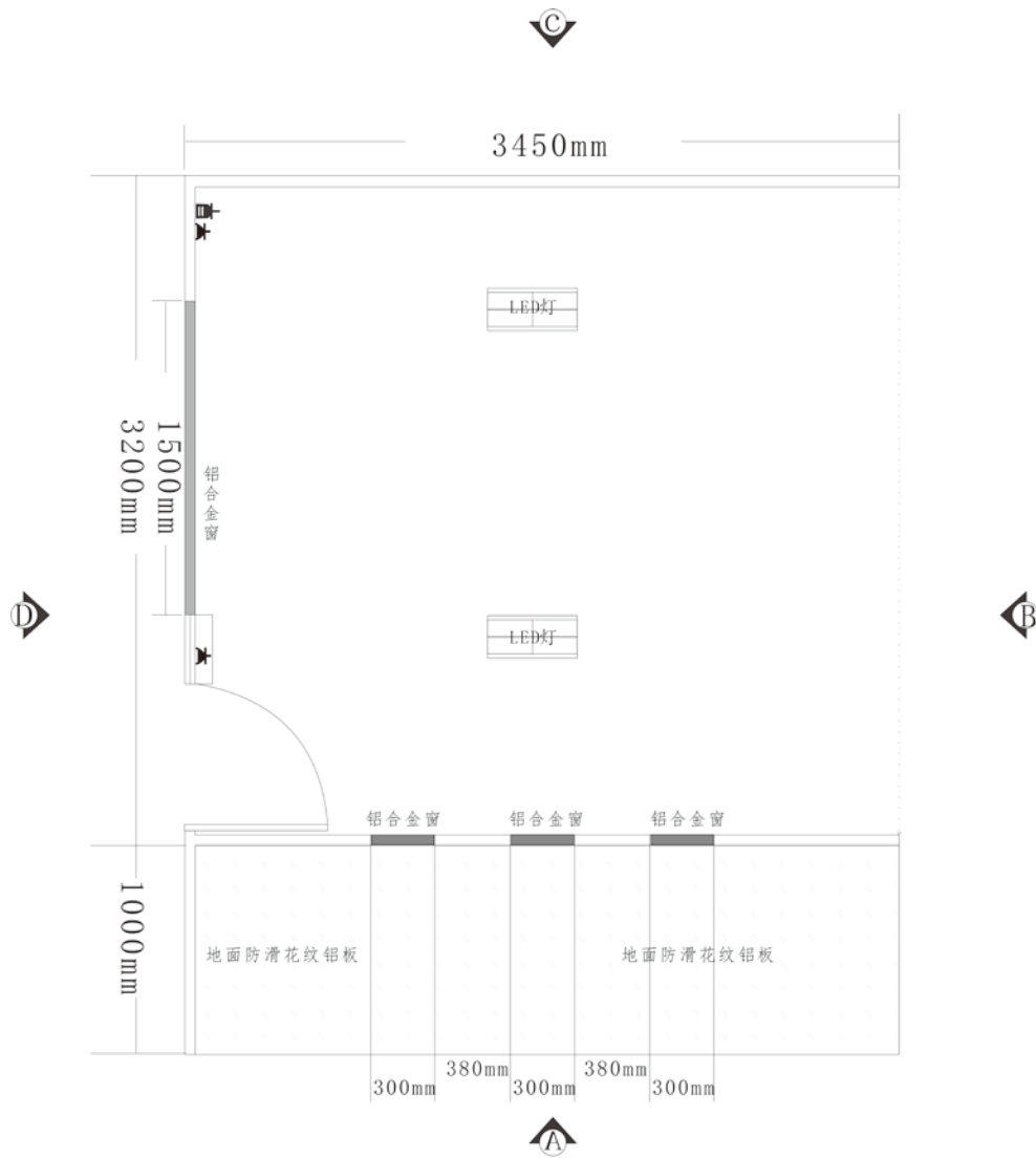
安全应急储备室平面图
